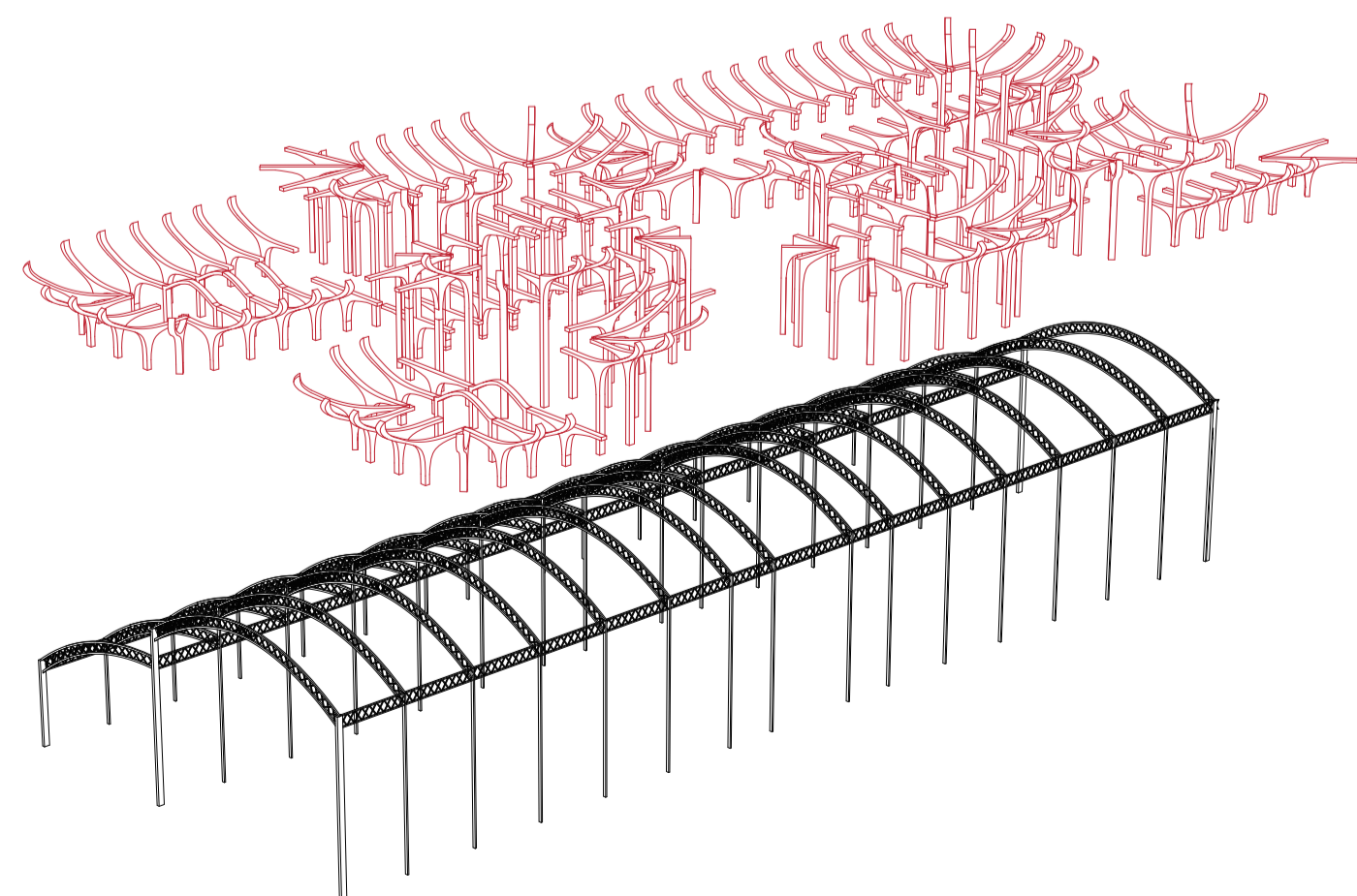
南側の既存骨格を壊し、新たな構造体としてプレキャストコンクリートを入れる。
